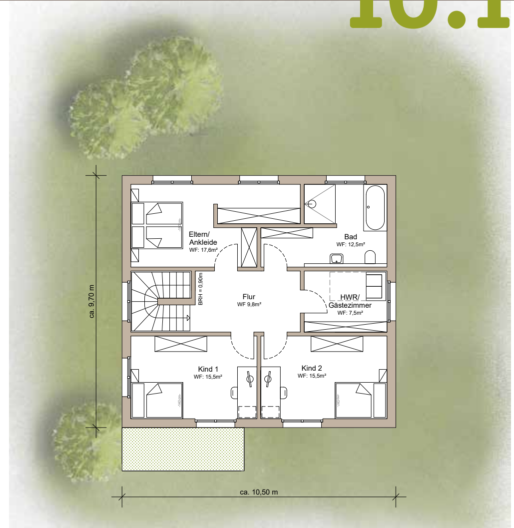
Obergeschoss WF: 78,4 m²
